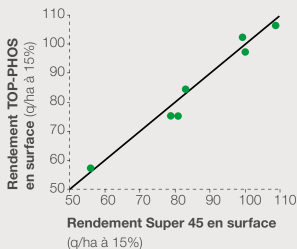
Figure 2 : rendements obtenus avec des apports de Top-Phos Duo M22 comparés à ceux obtenus avec des apports de Super 45. Les doses de phosphore sont identiques (40 kg P 2 O 5 /ha) et toujours apportées en surface, au semis de la céréale. Résultats de sept essais Arvalis de 2016 à 2018 (3 essais blé tendre, 4 essais blé dur, dans les départements 30, 32 et 41). Teneur en P 2 O 5 Olsen dans ces essais comprise entre 13 et 51 ppm, pH eau compris entre 7,7 et 8,7.
