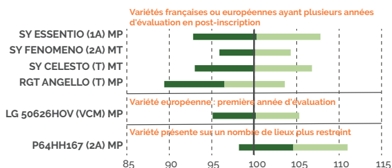
Figure 2 : 12 essais. Rendement moyen de la série : 37,3 q/ha. Indice de rendement (% de la moyenne des essais).
