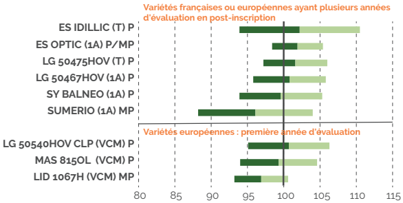
Figure 1 : 6 essais. Rendement moyen de la série : 39,9 q/ha. Indice de rendement (% de la moyenne des essais).
