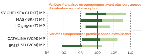
Figure 5 : 8 essais. Rendement moyen de la série : 38,1 q/ha. Indice de rendement (% de la moyenne des essais).
